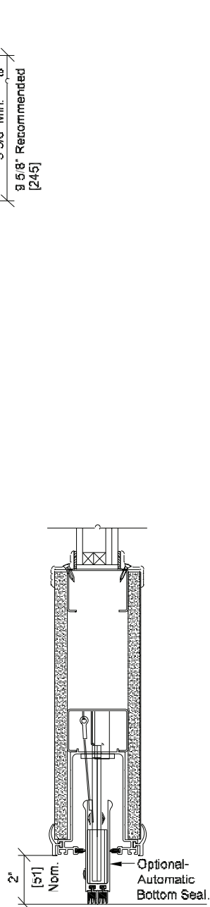
Optional Automatic Bottom Seal
